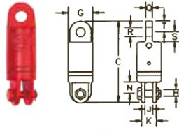
S-4 Øje/Gaffel S-4 Eye/Jaw
