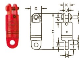
S-3 Gaffel/Øje S-3 Jaw/Eye
