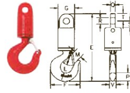
S-6 Øje/Krog S-6 Eye/Hook
