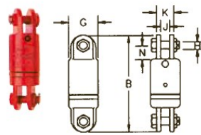
S-2 Gaffel/Gaffel S-2 Jaw/Jaw
