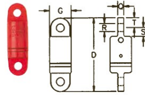
S-5 Øje/Øje S-5 Eye/Eye
