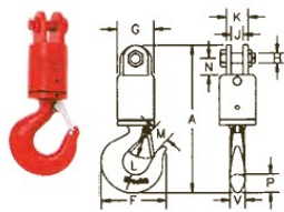
S-1 Gaffel/Krog S-1 Jaw/Hook
